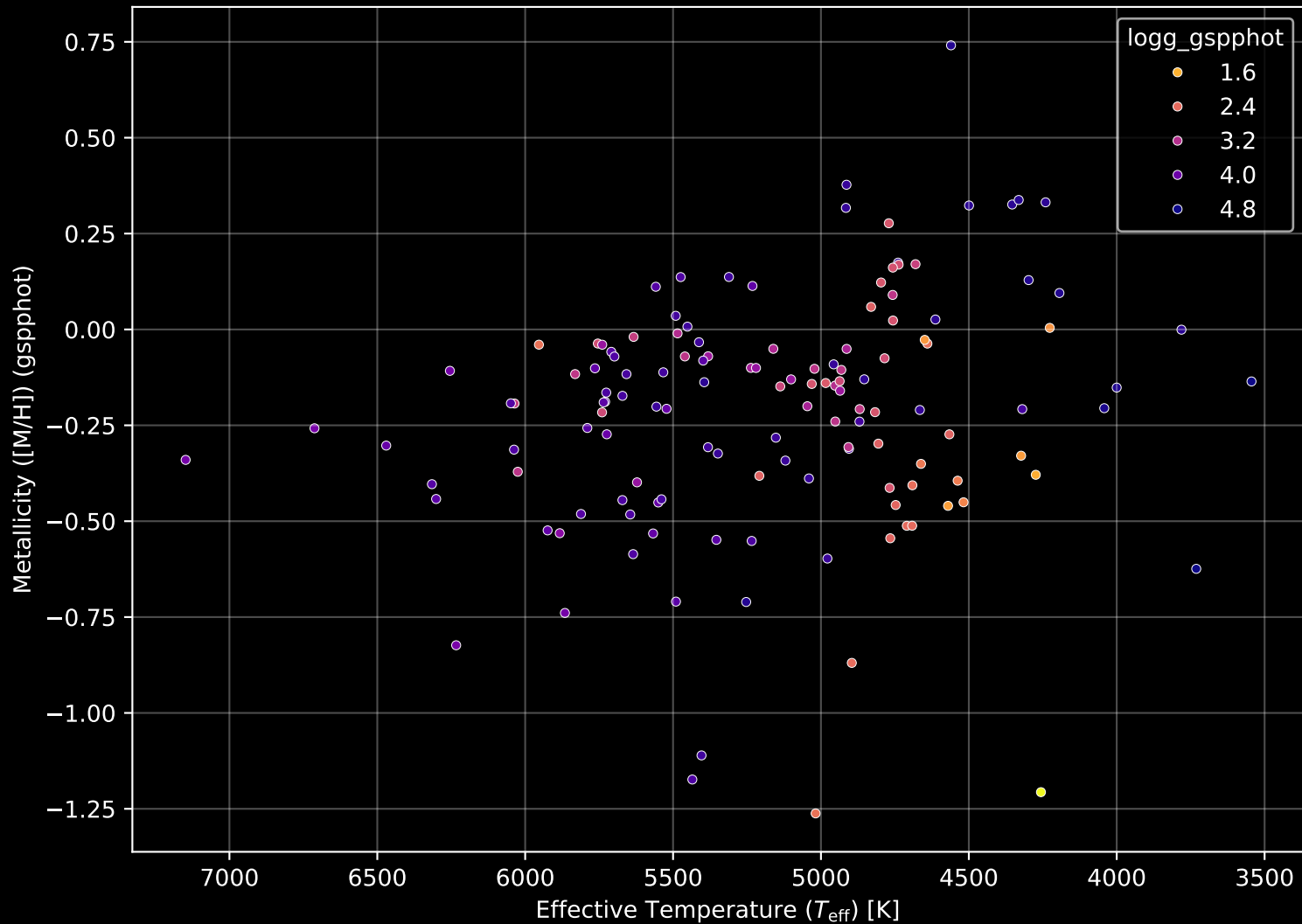
APOGEE DR17 Field: [042+45_MGA] Stellar Population Parameters (n= 135)
